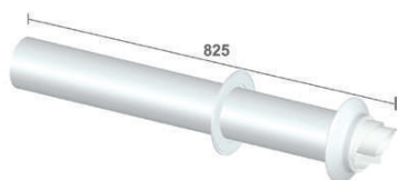
Horizontalni produžetak 60/100 , završni, 825 mm bez koljena
